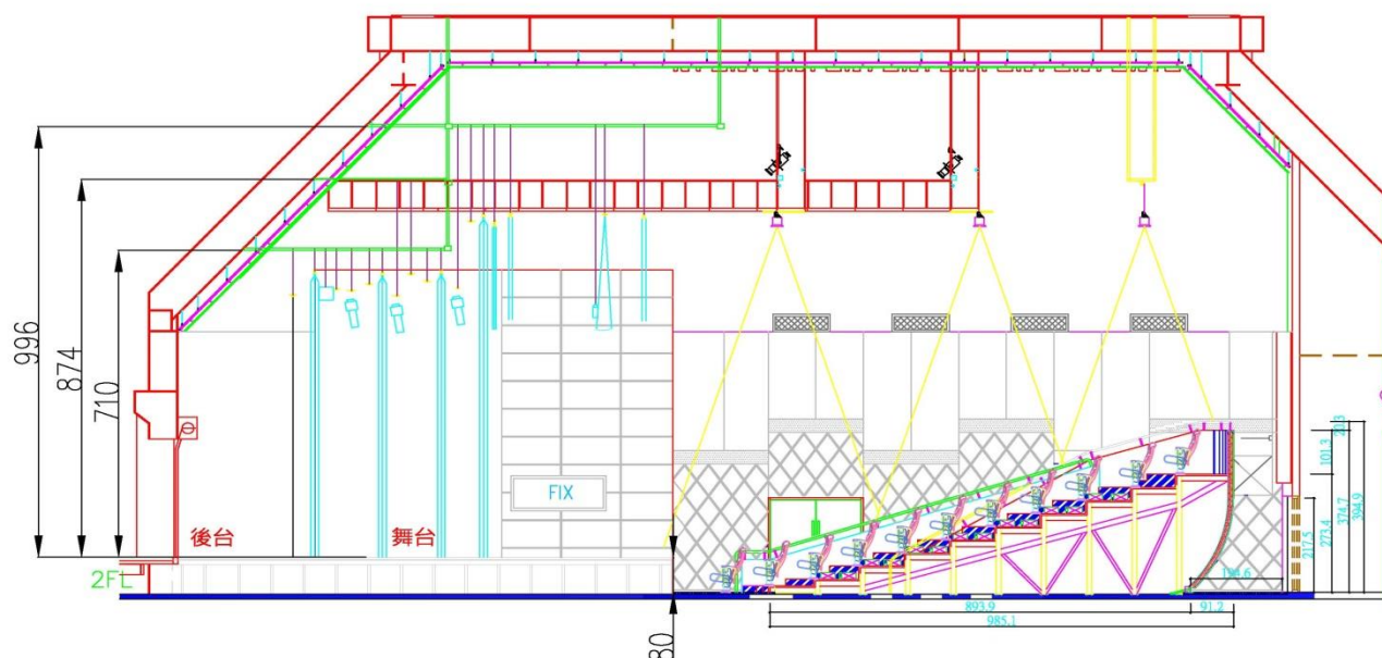
劇場剖面圖配置圖
