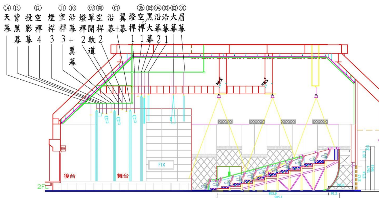
劇場吊桿剖面配置圖
